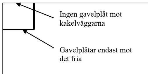
Figur 2. Exempel planritning montering kökskåpa mot vägg.
